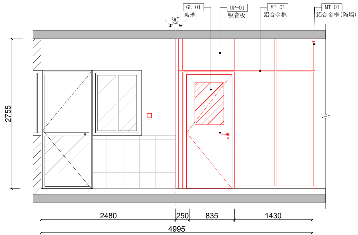
14 立面图 比例:1:40 #A3
