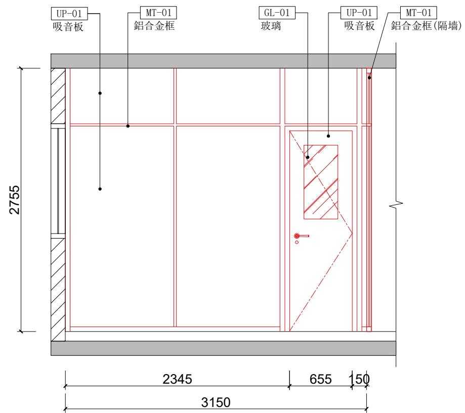
15 立面图 比例:1:40 #A3
