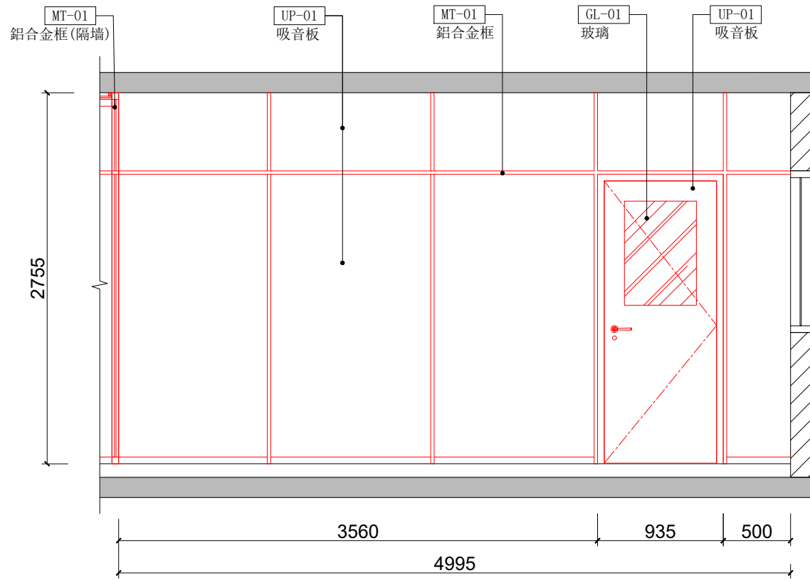
13 立面图 比例:1:40 #A3
