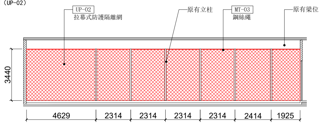
3 立面圖 比例: 1:120 @A3
