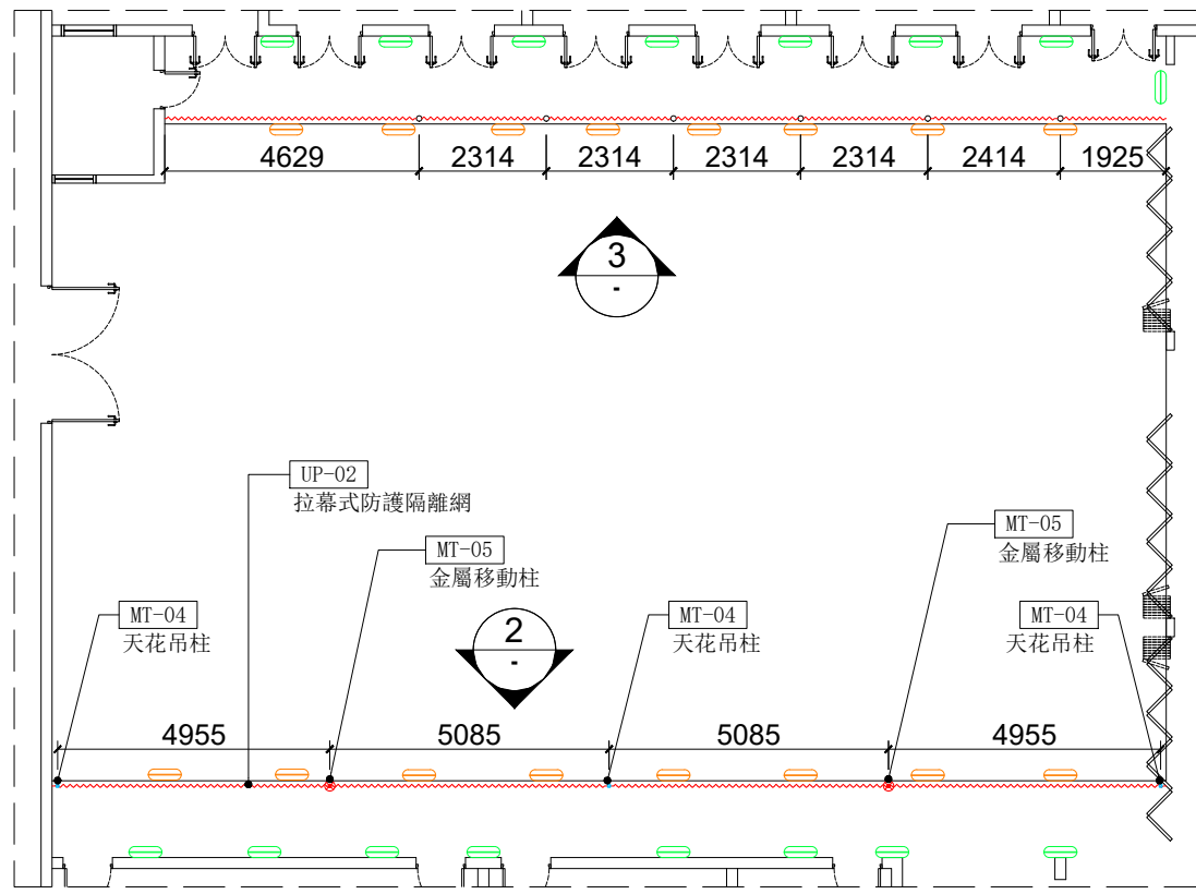
1 操場平面佈置圖 SCALE 1:150
