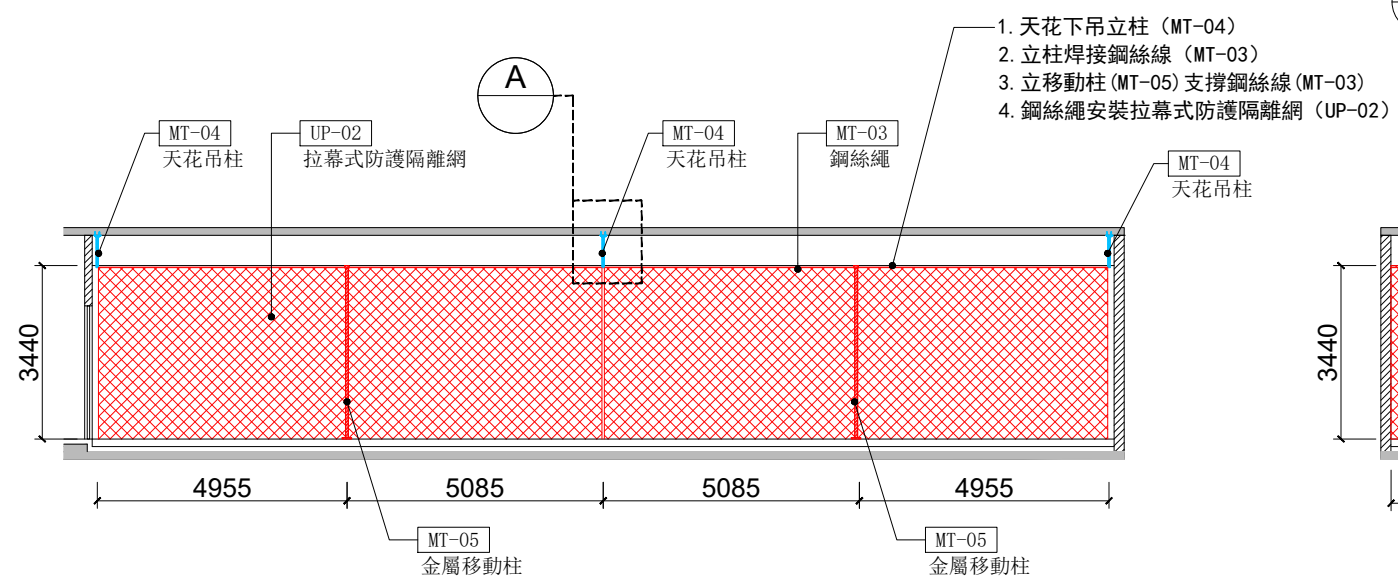
2 立面圖 比例: 1:120 @A3
